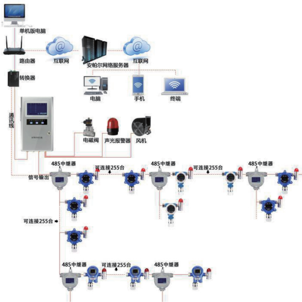
RS-485 通讯系统图
