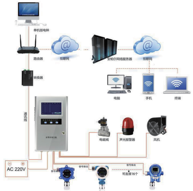
4-20MA 通讯系统图
